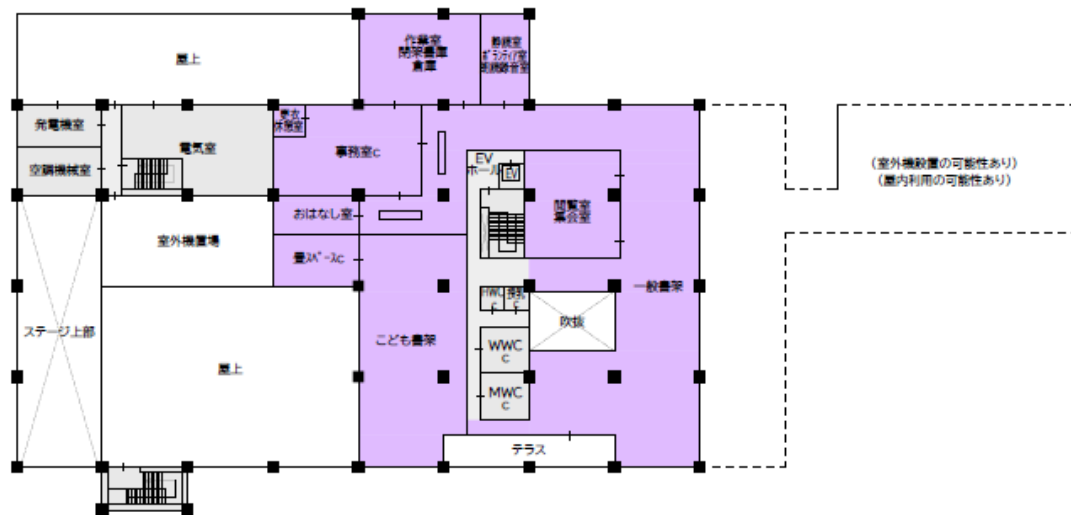
4階計画図
