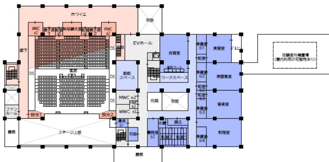
3 階計画図
