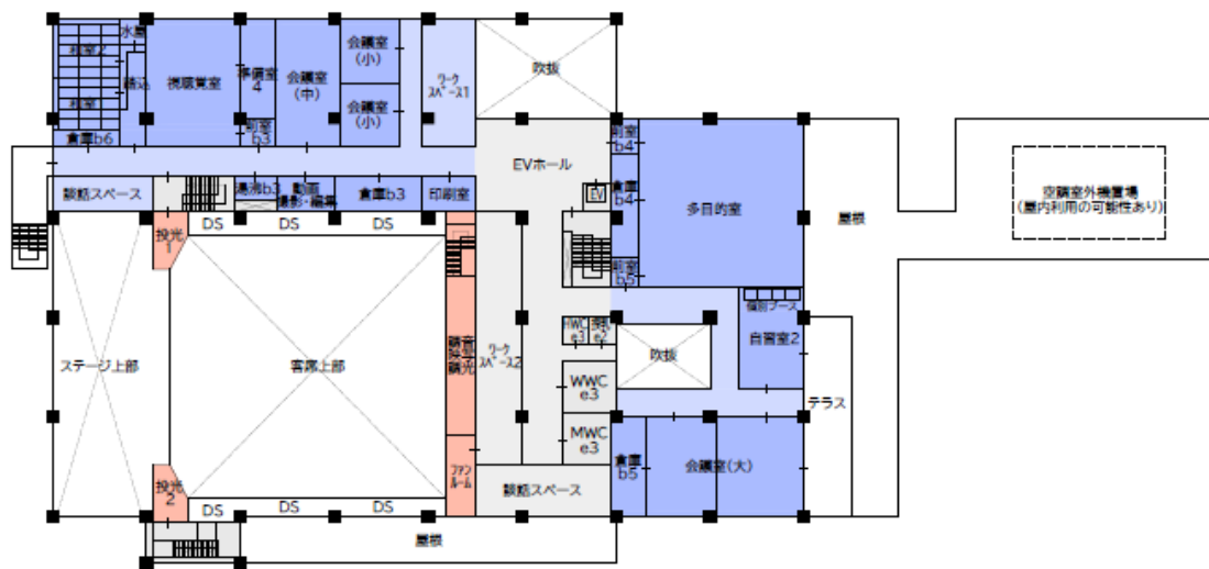
3階計画図
