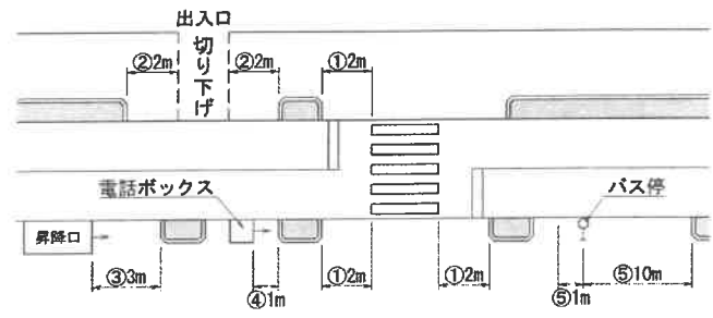
図Ⅲ-2 植樹帯設置を避けるべき範囲
