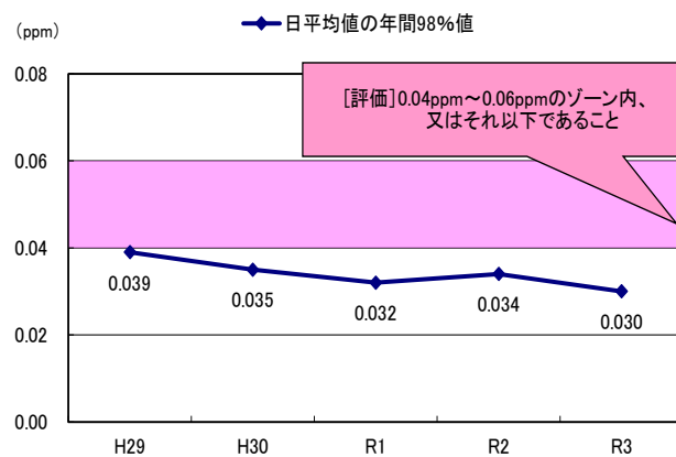
図 3-2 二酸化窒素濃度の推移
