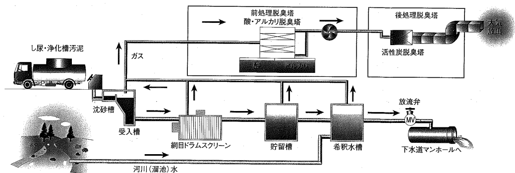
図 3-18 処理フロー
