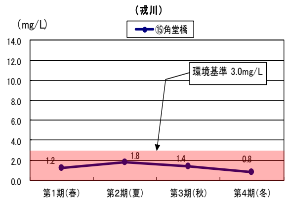
図 3-9 令和 3 年度 BOD の季節変動
