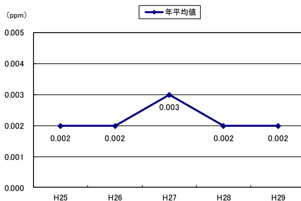
図 3-1 二酸化硫黄濃度の推移
