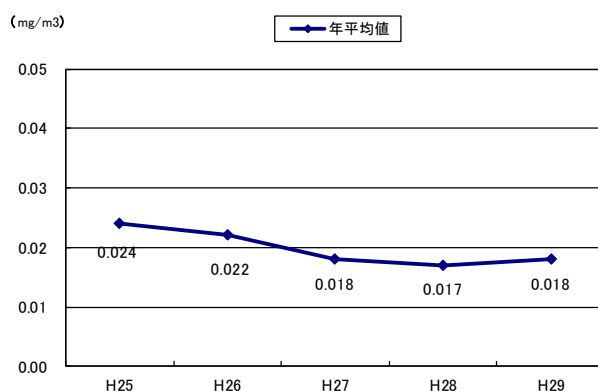
図 3-3 浮遊粒子状物質濃度の推移
