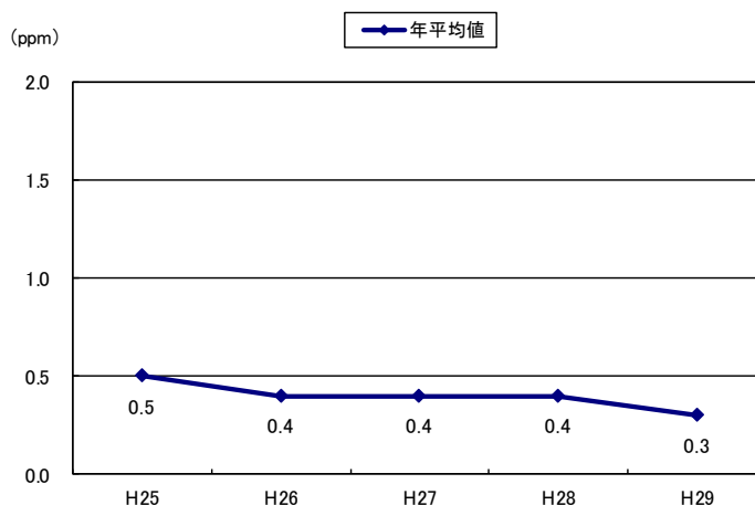
図 3-4 一酸化炭素濃度の推移
