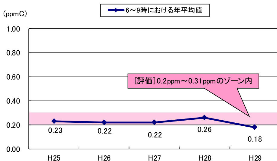
図 3-5 非メタン炭化水素濃度の推移
