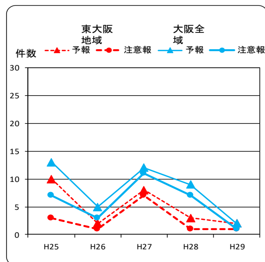
図 3-7 光化学スモッグ予報等の発令件数推移
