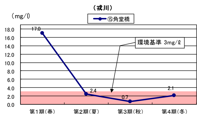
図 3-9 平成 29 年度 BOD の季節変動
