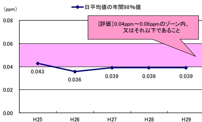
図 3-2 二酸化窒素濃度の推移
