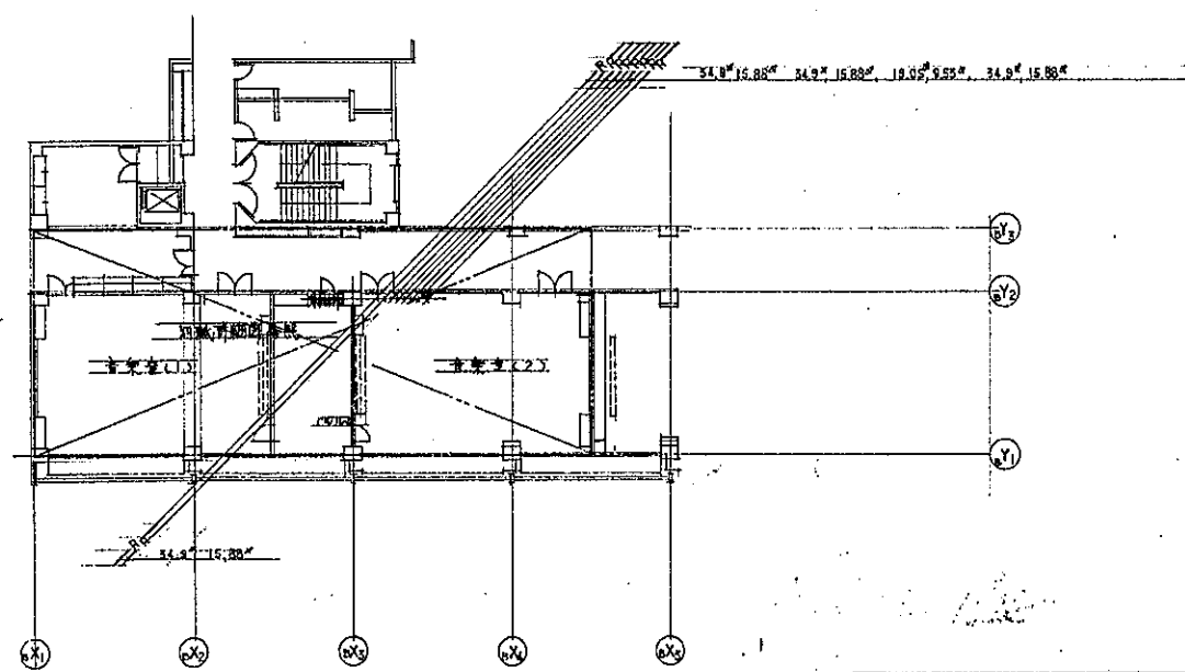
4 楼平面图 1:200
