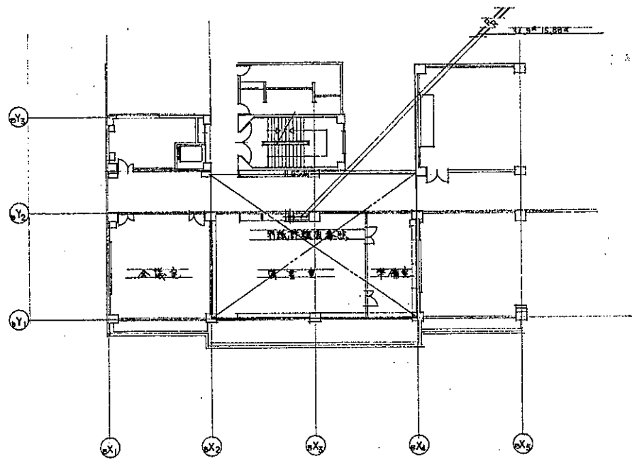
2 楼平面图 1:200
