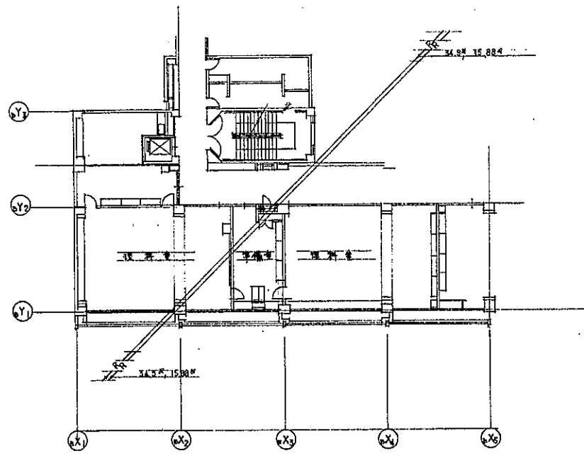
3 楼平面图 1:200
